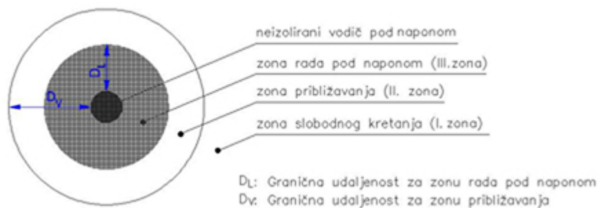
Slika 1. Zona rada pod naponom i zona približavanja
