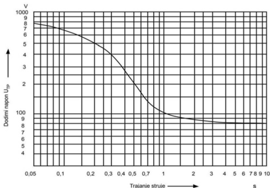
Slika 7. Dijagram dopušćenog dodirnog napona u odnosu na vrijeme trajanja struje
