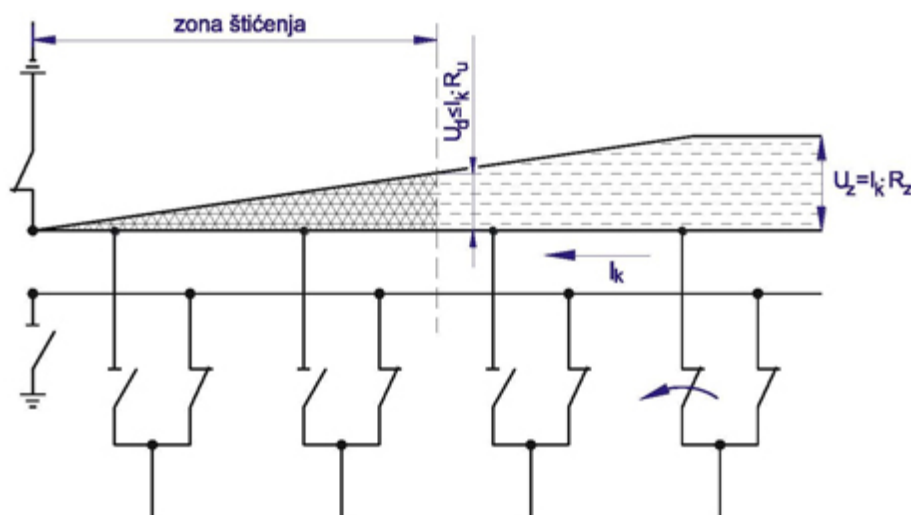
Slika 6. Zona šticeanja uzemljivača
